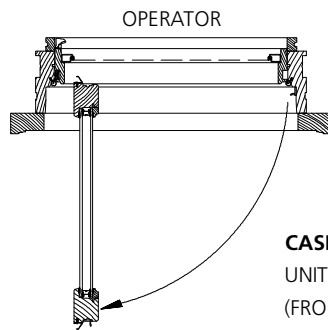
LEFT HAND
