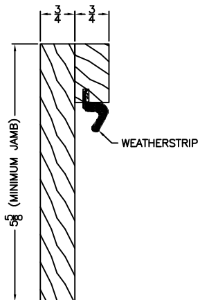
SIDE JAMB PROFILE
