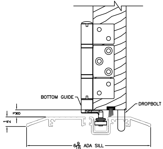
ADA SILL (Available Upon Request)
