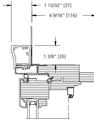
BRICKMOULD
