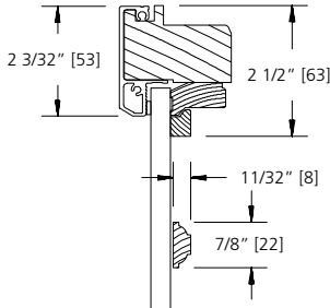
7/8" GRILLE BAR
