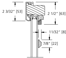
7/8" GRILLE BAR
