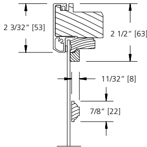
7/8" GRILLE BAR
