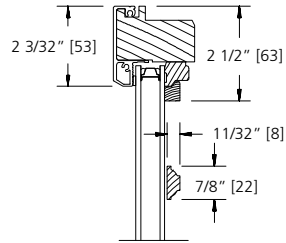
7/8" GRILLE BAR
