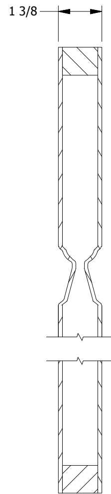
SECTION A-A
