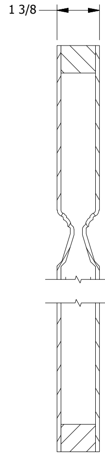
SECTION A-A
