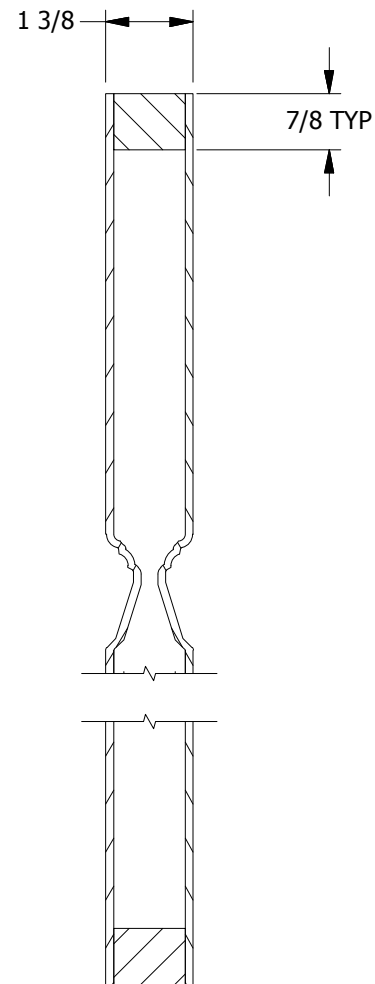
SECTION A-A
