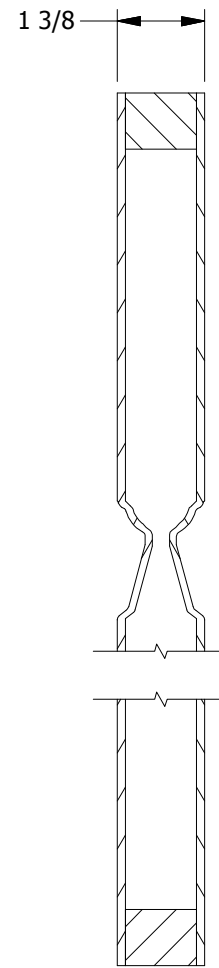
SECTION A-A
