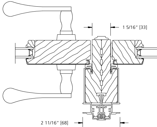
SIDE JAMB
