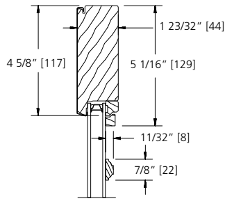
7/8" GRILLE BAR
