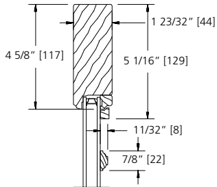
7/8" GRILLE BAR
