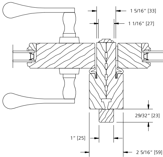
SIDE JAMB
