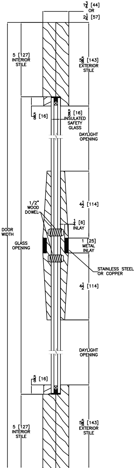
HORIZONTAL DOOR CROSS SECTION
