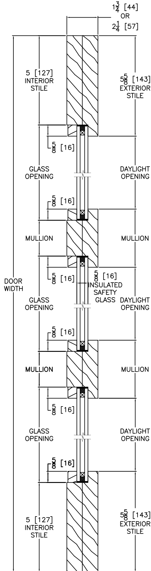
HORIZONTAL DOOR CROSS SECTION
