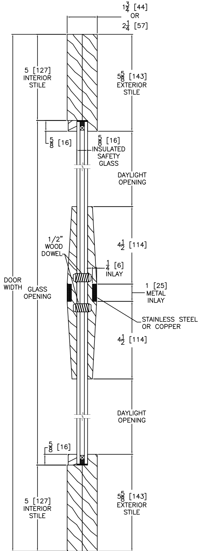
HORIZONTAL DOOR CROSS SECTION
