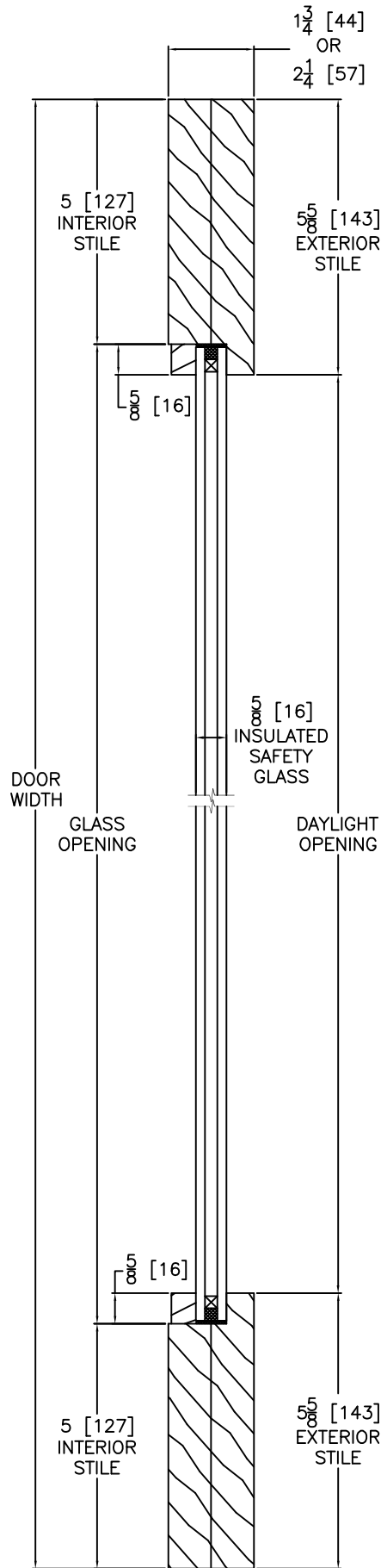
HORIZONTAL DOOR CROSS SECTION
