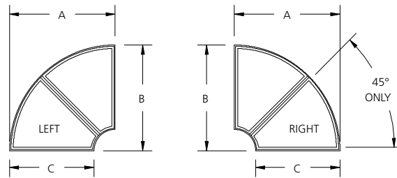
TYPE DI - 2 TYPE EI - 2 INVERTED QUARTER ROUND - TWIN
