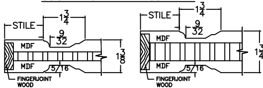
OG STICKING WITH "D1" DOUBLE HIP
